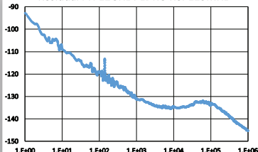
Residual PN 12GHz PLDRO Ref 125MHz
